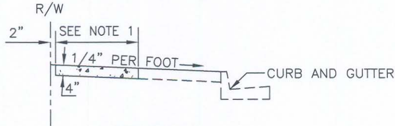
SECTION N.T.S.
